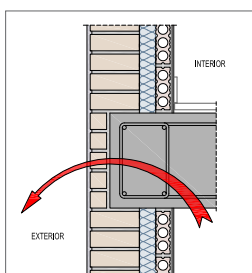
Puente térmico cuando el aislamiento está por el interior.
