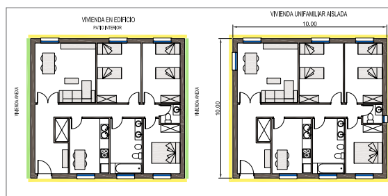
Figura 6. Afectación puentes térmicos en función de la tipología de vivienda.
